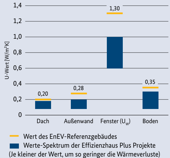
Abbildung 23: Wärmedurchgangskoeffizienten
