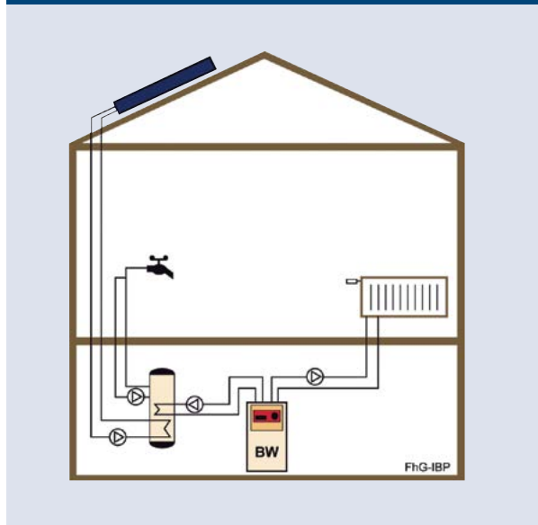
Abbildung 11: Schematische Darstellung einer Heizanlage mit solarer Warmwasserbereitung
